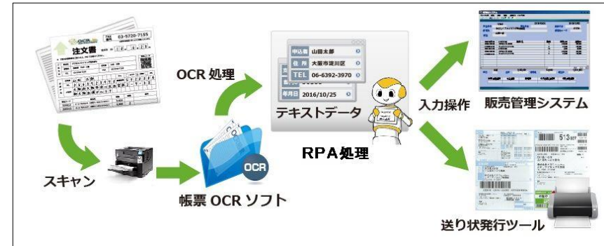
OCR+RPA連携図
